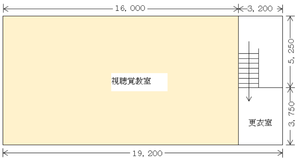
第二教棟 1 階
