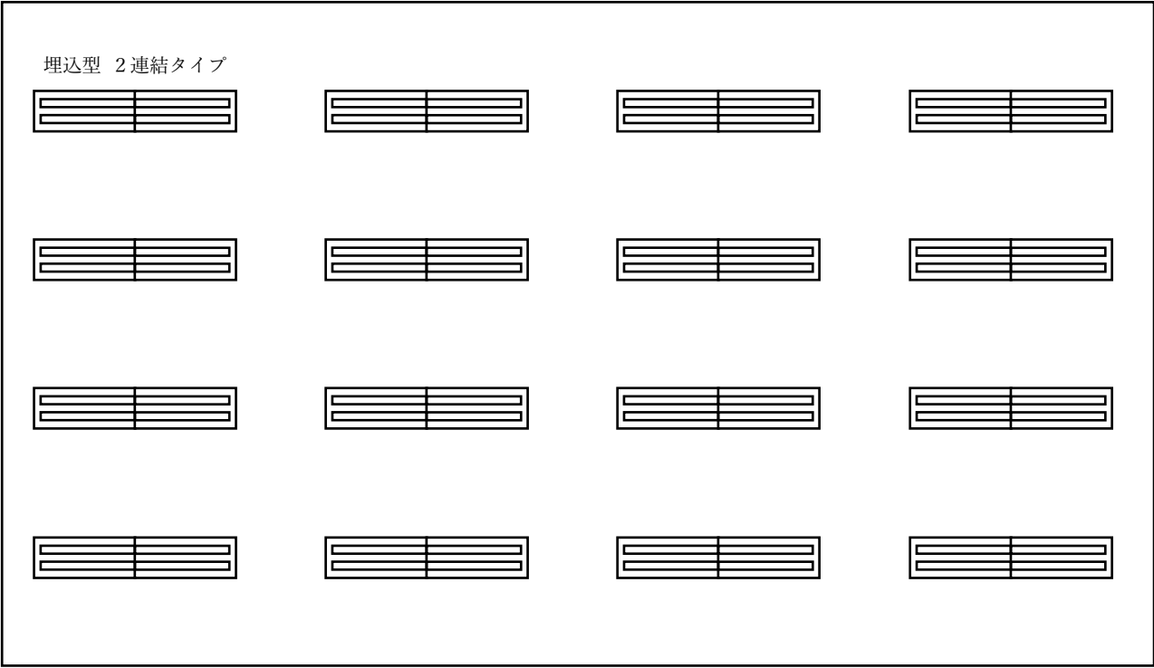
1 階視聴覚教室 平面図(天井)
