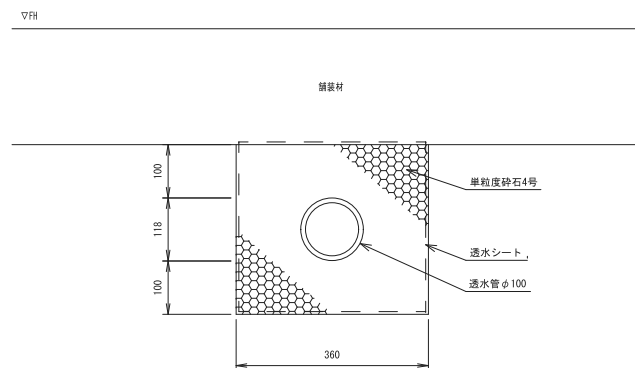
透水管断面図 S=1:10
