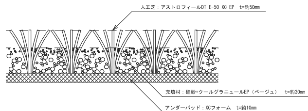
ロングパイル人工芝詳細図 S=1:3
