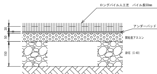
ロングパイル人工芝舗装断面図 S=1:10
