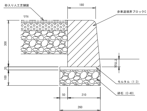
舗装止縁石-1詳細図 S=1:10
