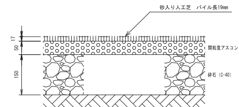
砂入り人工芝舗装断面図 S=1:10
