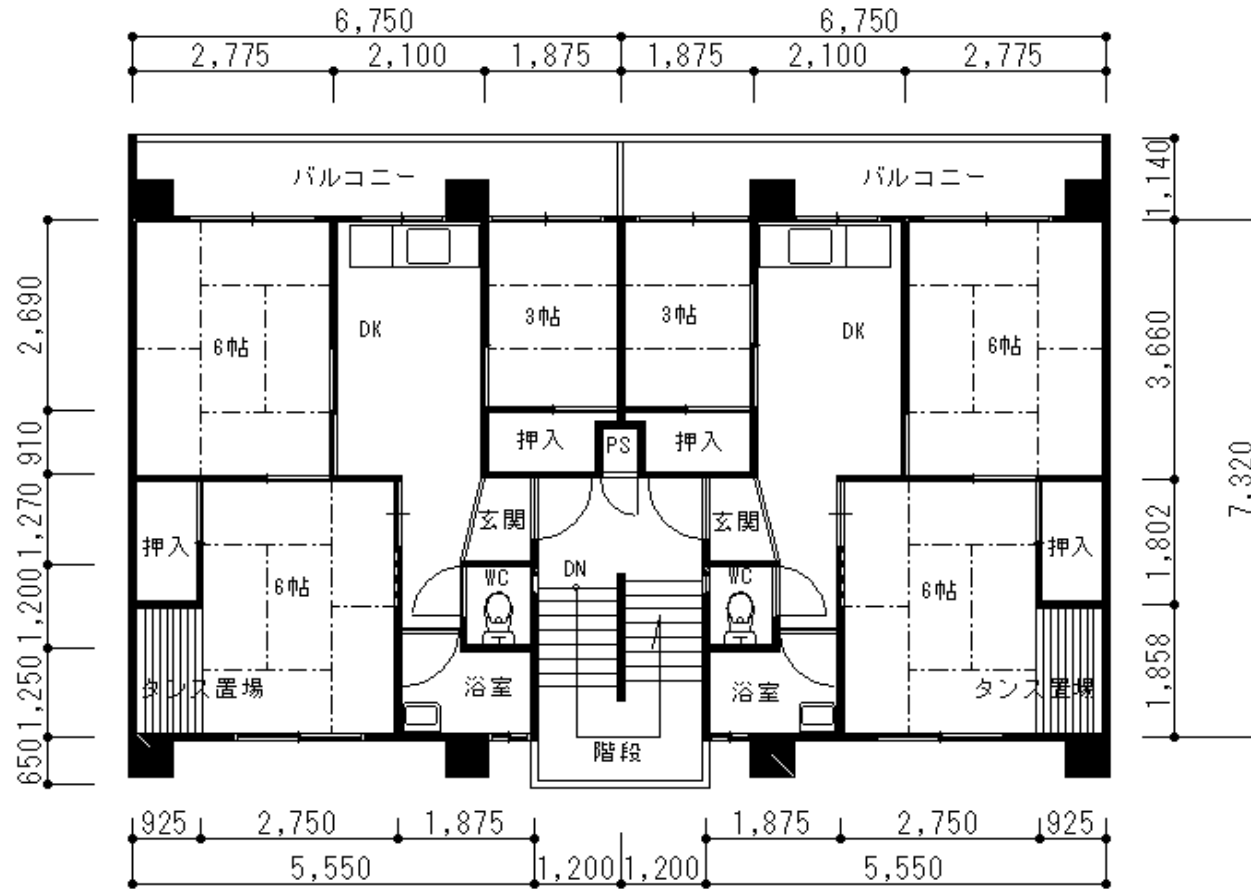
唐子団地 1・2号棟 平面図 S=1/100
