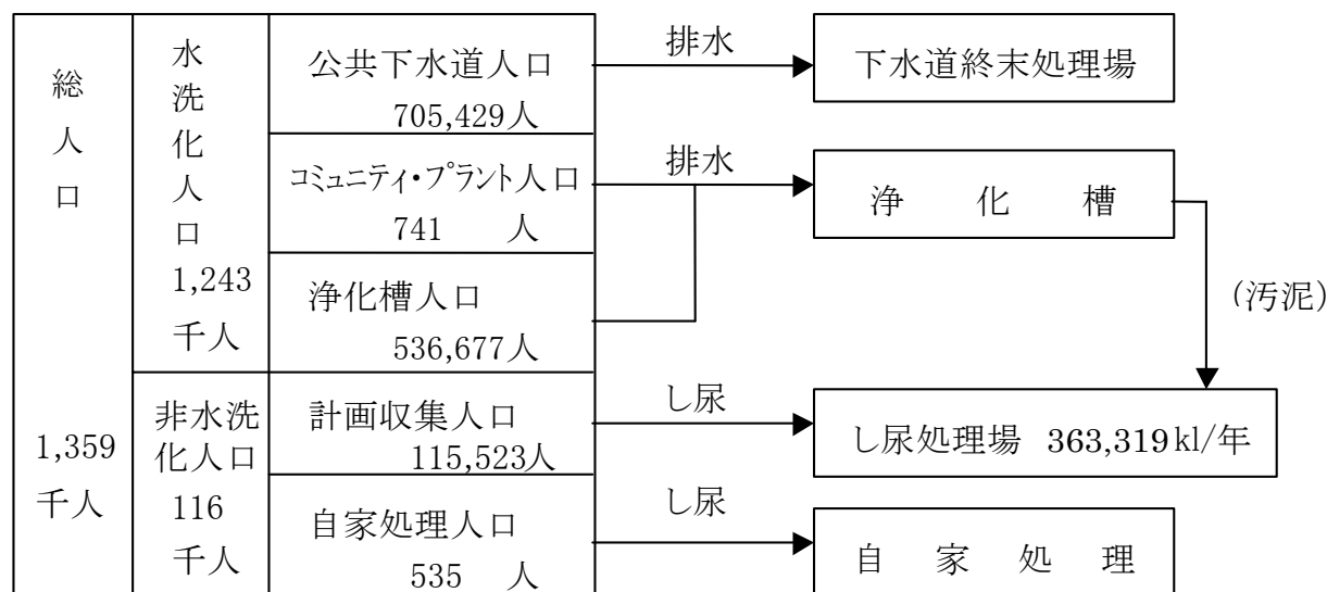
図2-3-2 し尿処理の状況(令和2年度)
