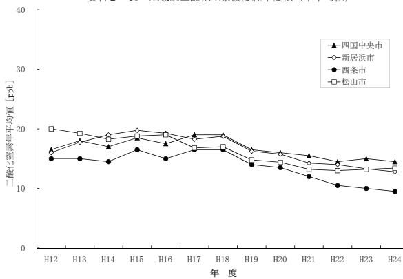
資料 2-16 地域別二酸化窒素濃度経年変化（年平均値）
