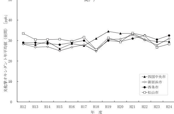
資料 2-17 地域別光化学オキシダント濃度経年変化（年平均値（昼間））
