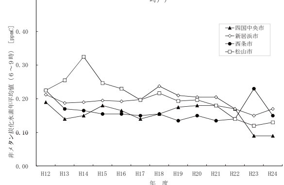
資料 2-18 地域別非メタン炭化水素濃度経年変化（年平均値（6～9時））
