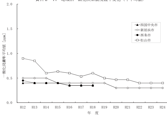
資料 2-14 地域別一酸化炭素濃度経年変化（年平均値）
