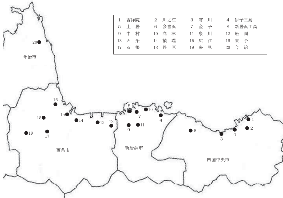
資料 2-4 大気汚染常時監視測定局配置図
