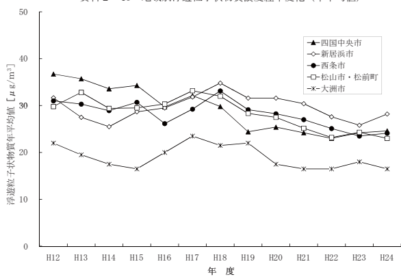
資料 2-15 地域別浮遊粒子状物質濃度経年変化（年平均値）
