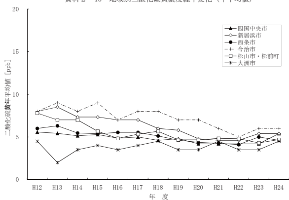
資料 2-13 地域別二酸化硫黄濃度経年変化（年平均値）
