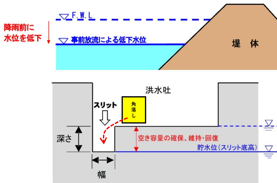
図 7.4. 既存ため池の事前放流と低水管理運用ルールの変更イメージ
