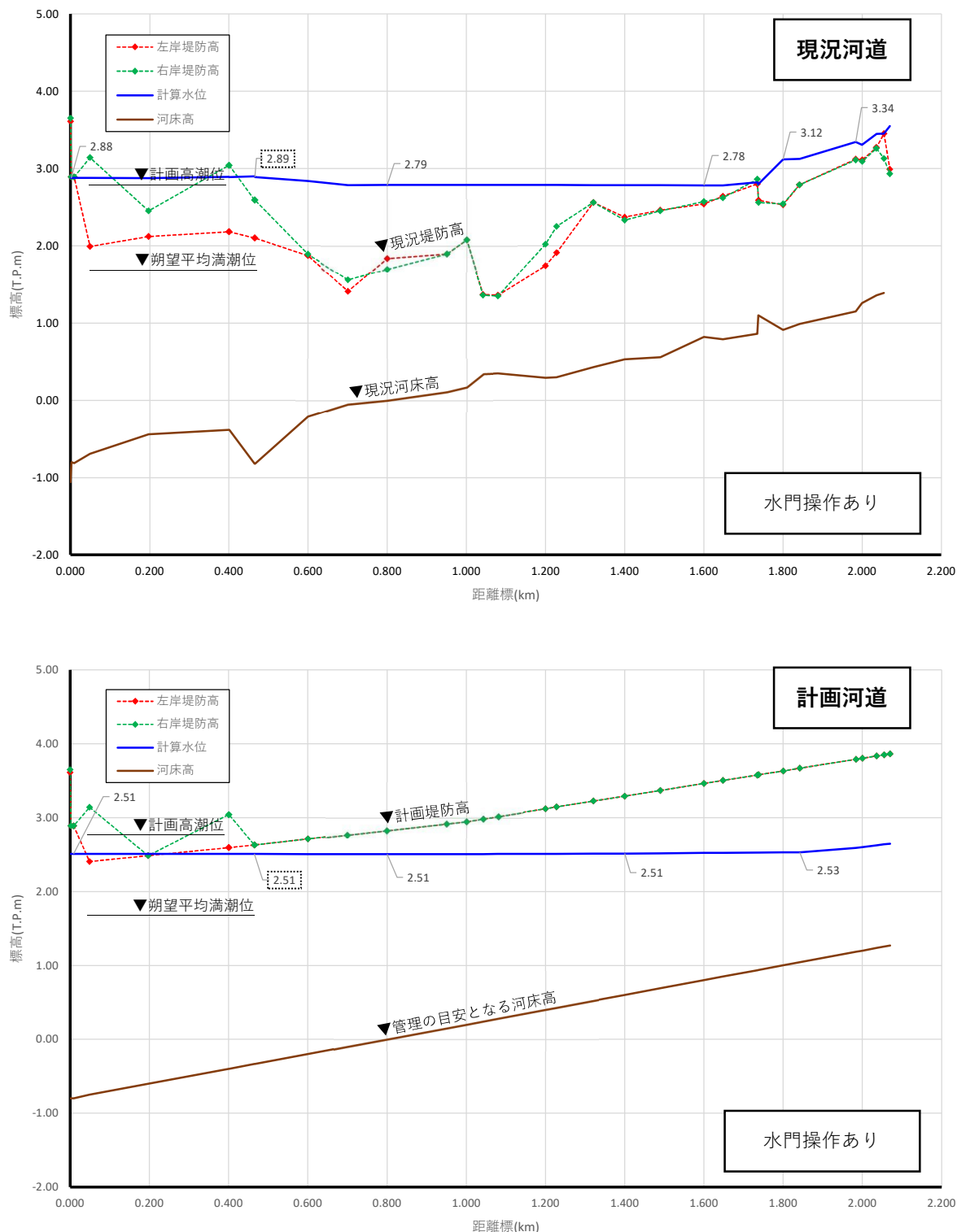
図 3.2. 計画対象降雨における都市浸水想定ピーク水位縦断図（現況河道及び計画河道）
