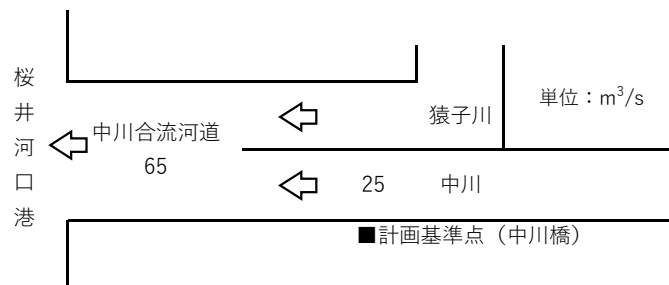
図 4.3. 中川水系計画高水流量配分図
