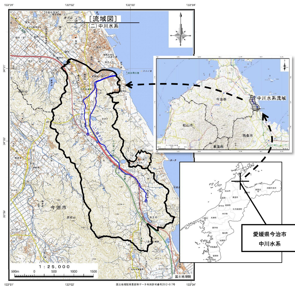
図 1.1. 中川流域図
