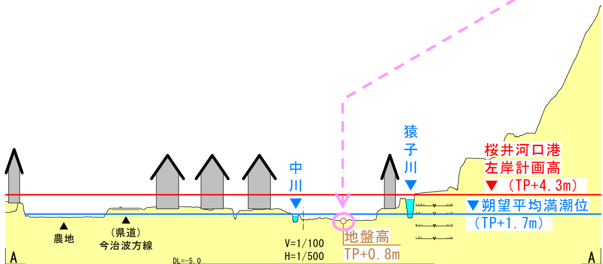
図 1.3. A - A 断面図 (河川流下方向) (林野庁作成公共測量成果 (H30) : 0.5m グリッドデータより横断面図を作成)
