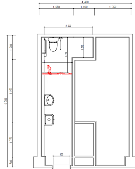
改修後 1階便所配置図
