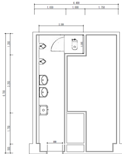
改修前 1階便所配置図
