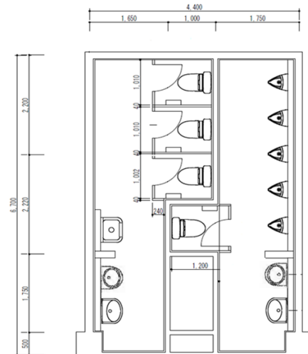
改修後 3階便所配置図
