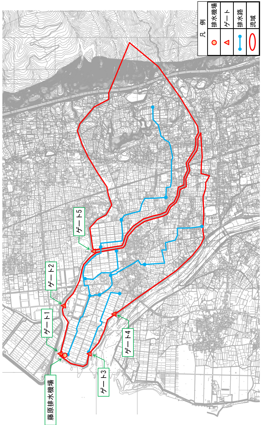
現況排水系統図
