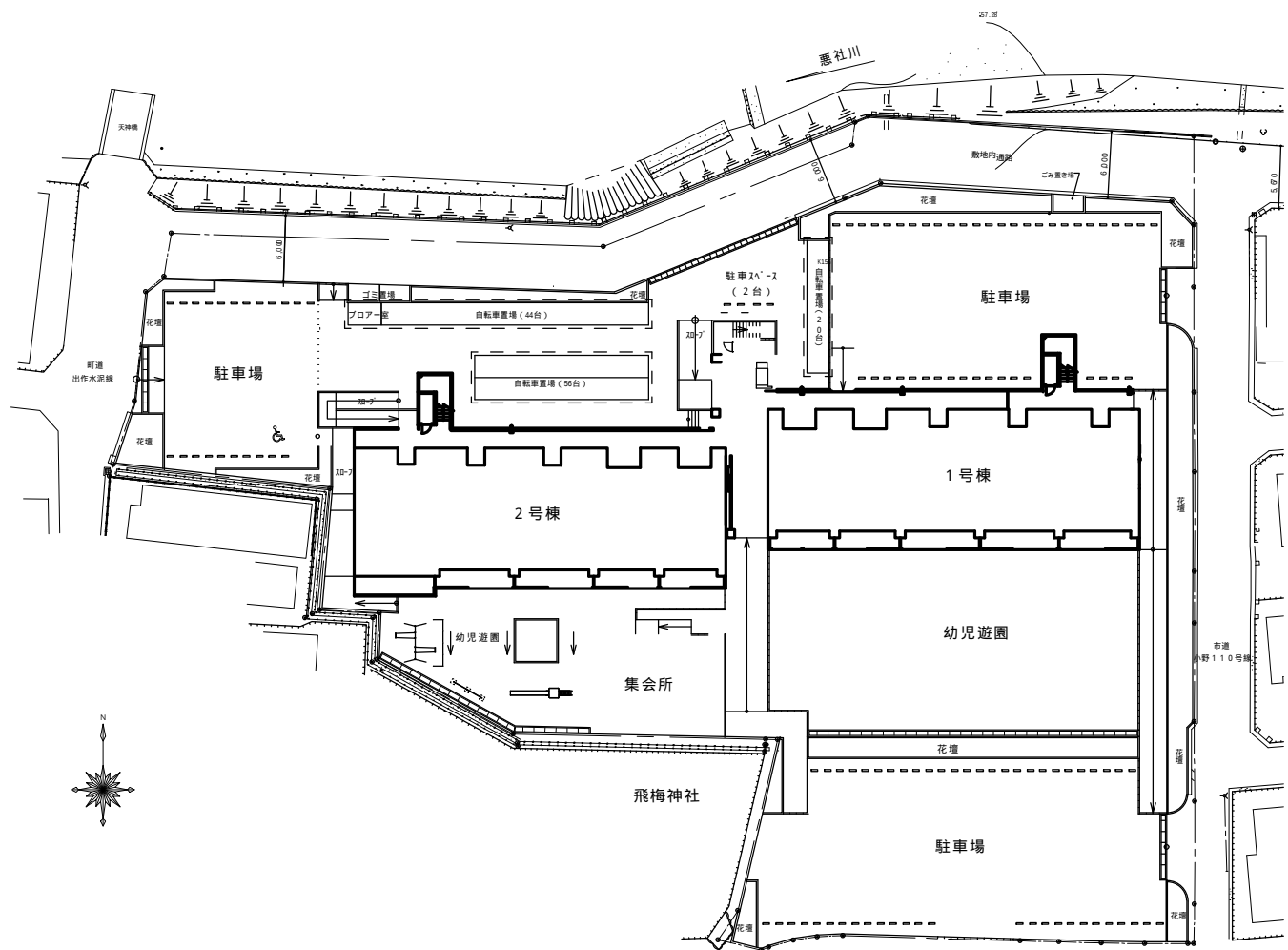
天神梅本団地 配置図 NonScale
