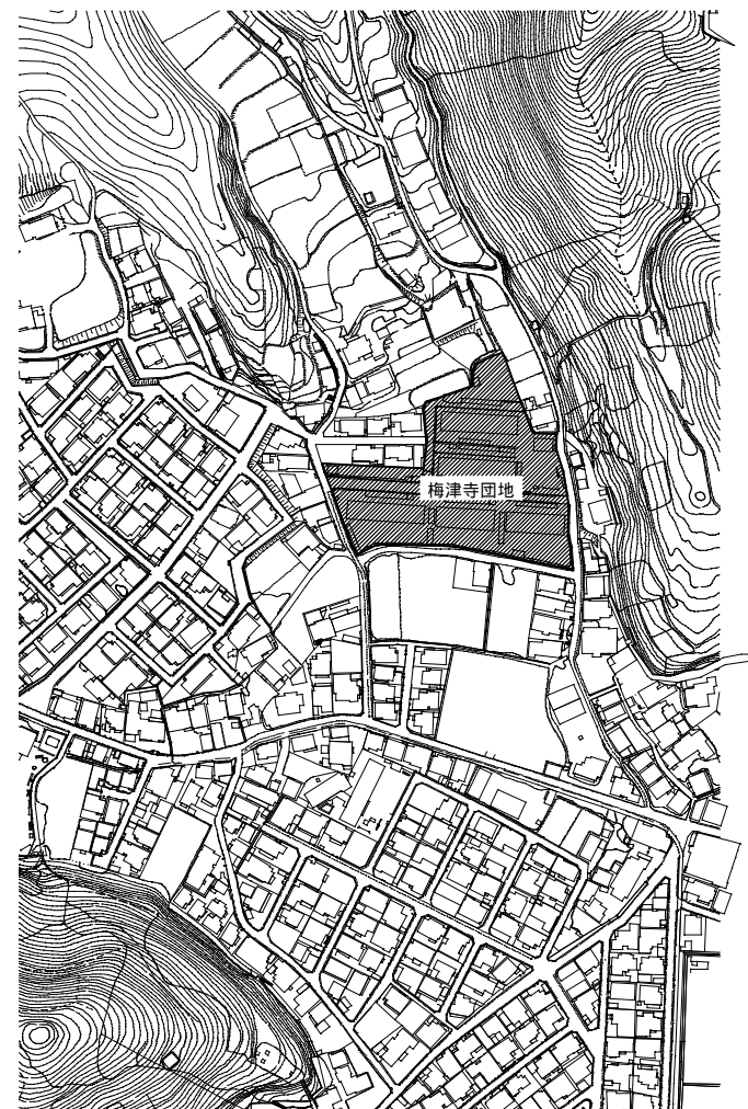
梅津寺団地 敷地案内図 NonScale
