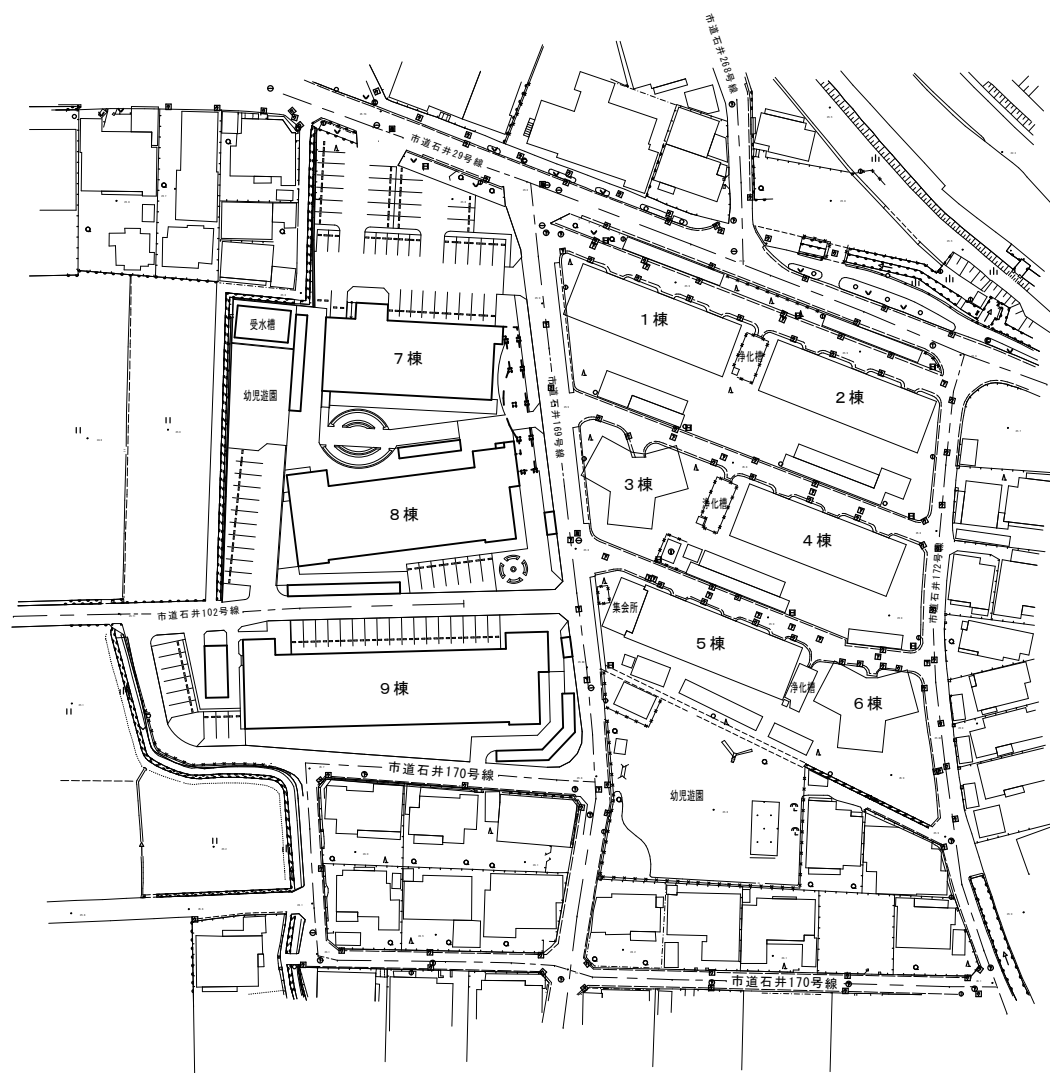
石井団地 配置図 NonScale
