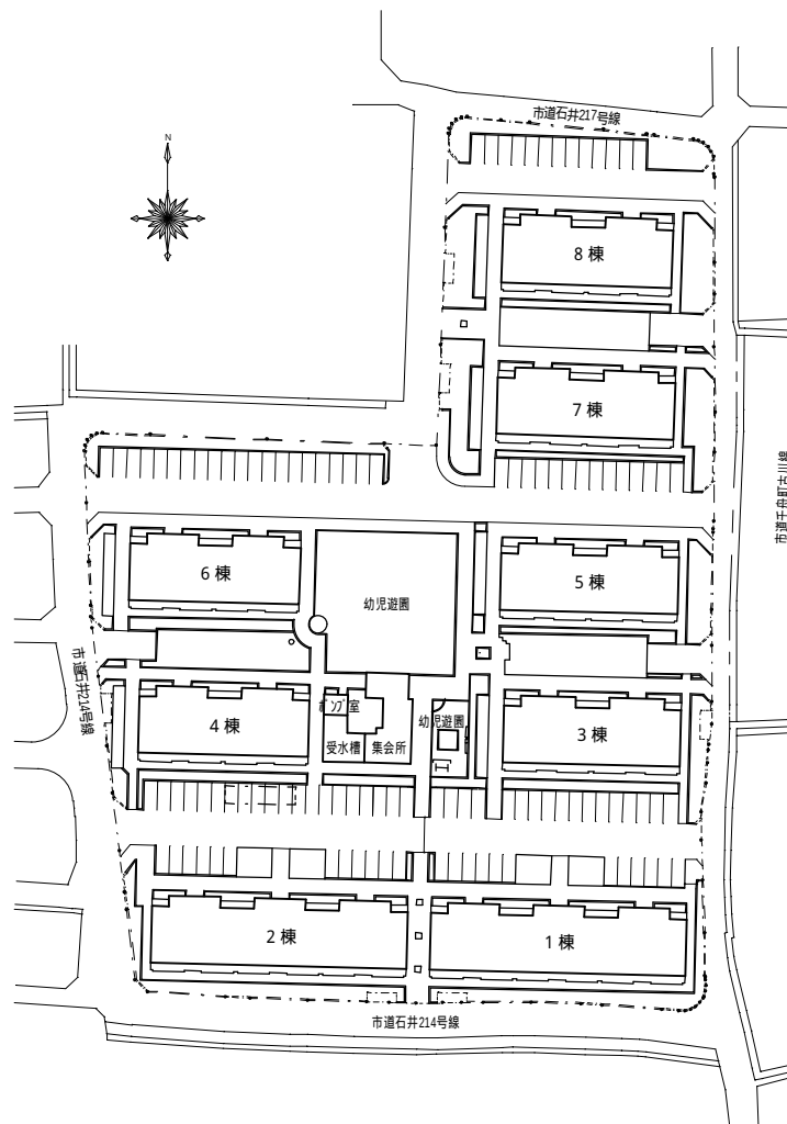
和泉団地 配置図 S : 1/500
