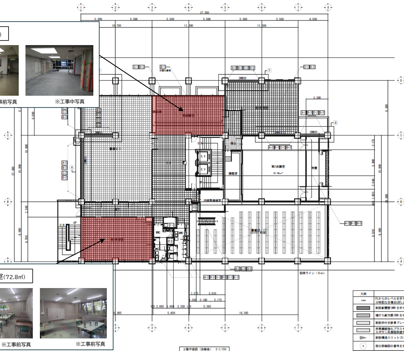
2階平面図(改修後) S:1/150
