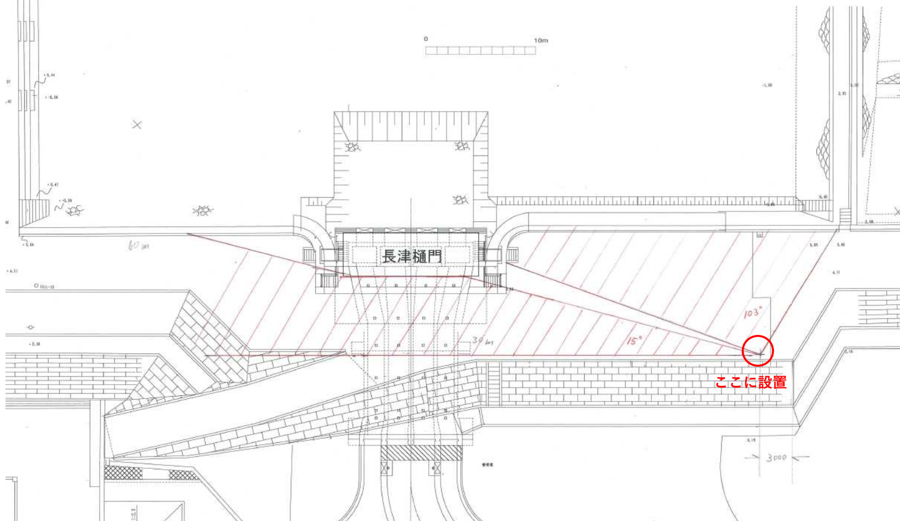
全体計画平面図 S=1:200
