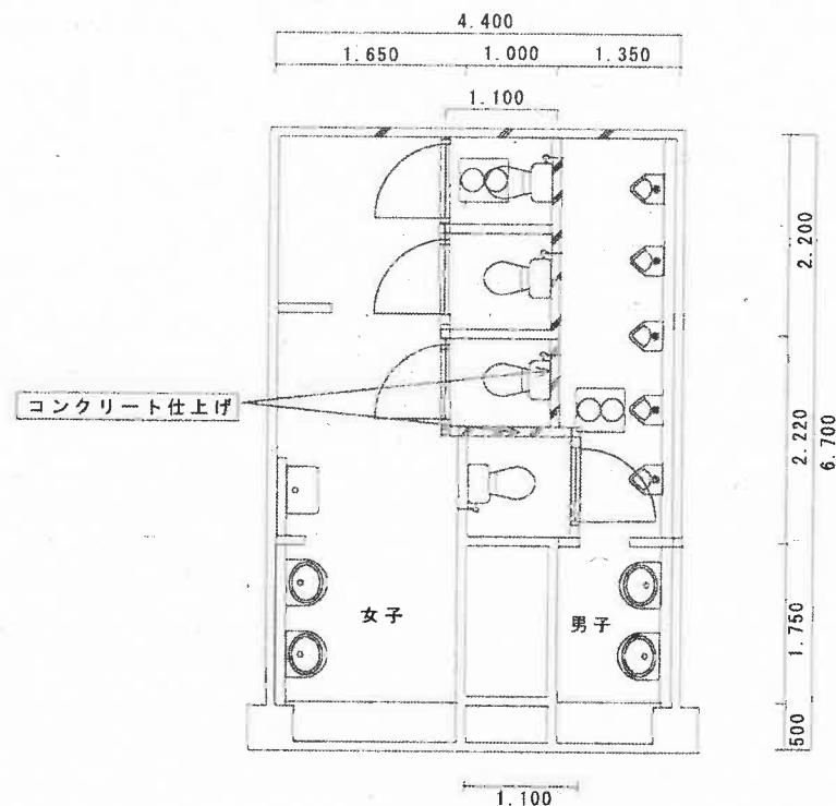
改修後2階便所配置図
