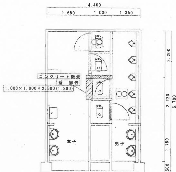
改修前2階便所配置図
