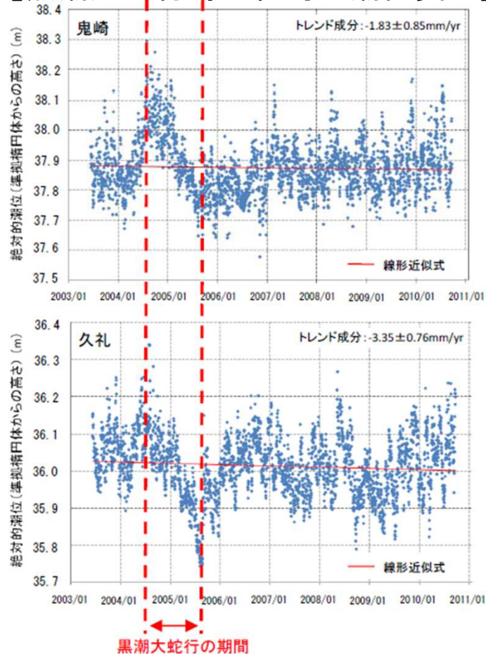
【黒潮大蛇行時の絶対的潮位変化】
