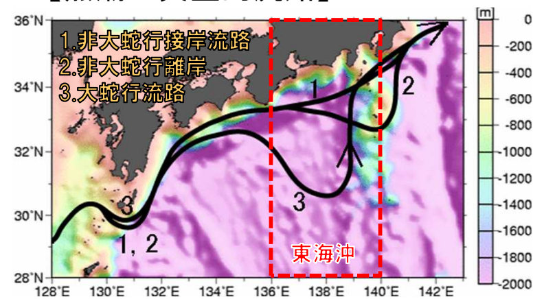
【黒潮の典型的流路】
