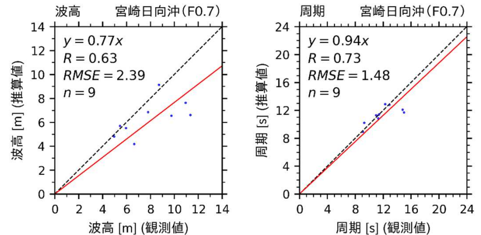
図2: 相関解析(宮崎日向沖、 F=0.7 )
