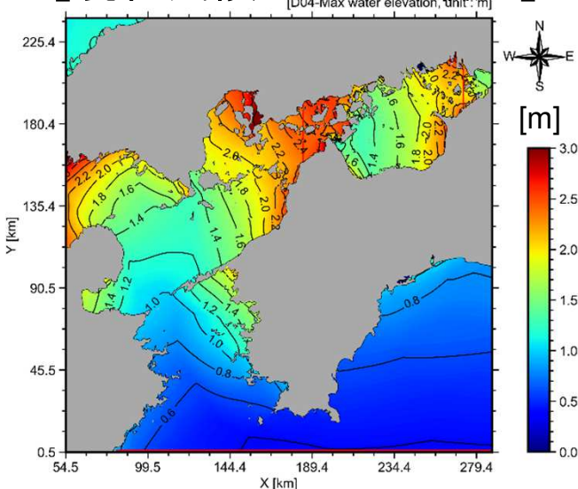
【現在気候:8コース最大】
