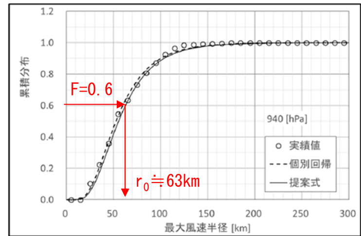
図：本多モデルによる r_0 の分布
