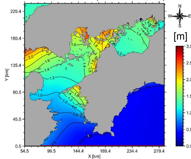
【将来気候:8コース最大】
