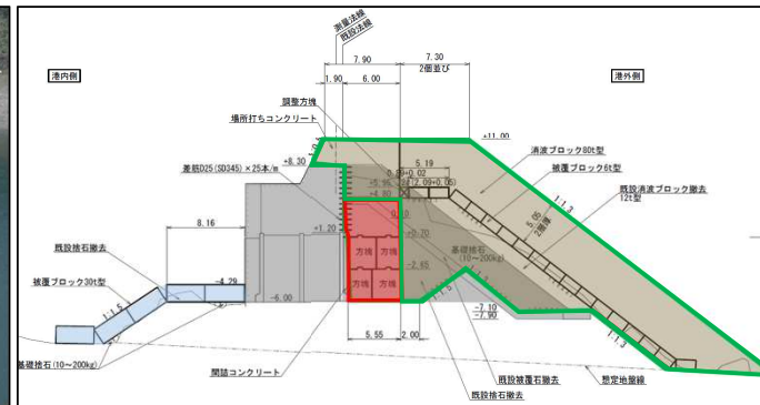
第一防波堤（R3～）
