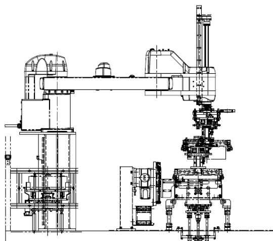
水平多関節ROBO
