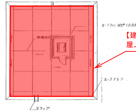
屋上平面図
