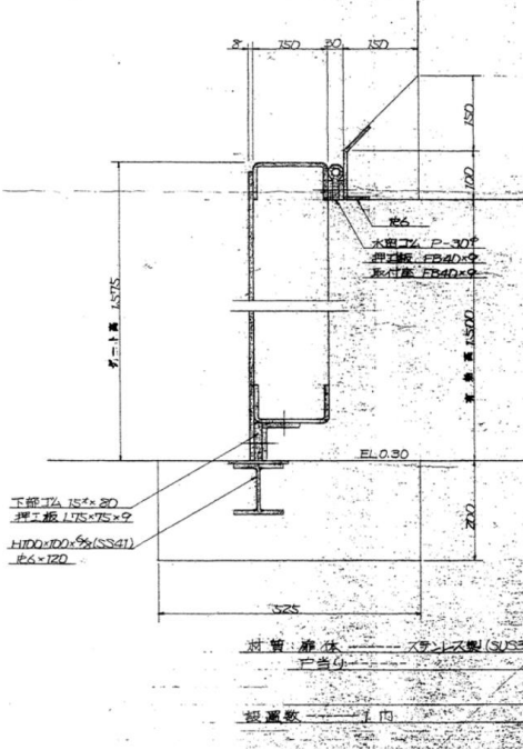
上下部詳細図 S-1
