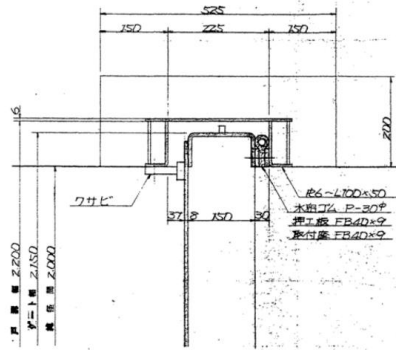
上下部詳細図 S-1
