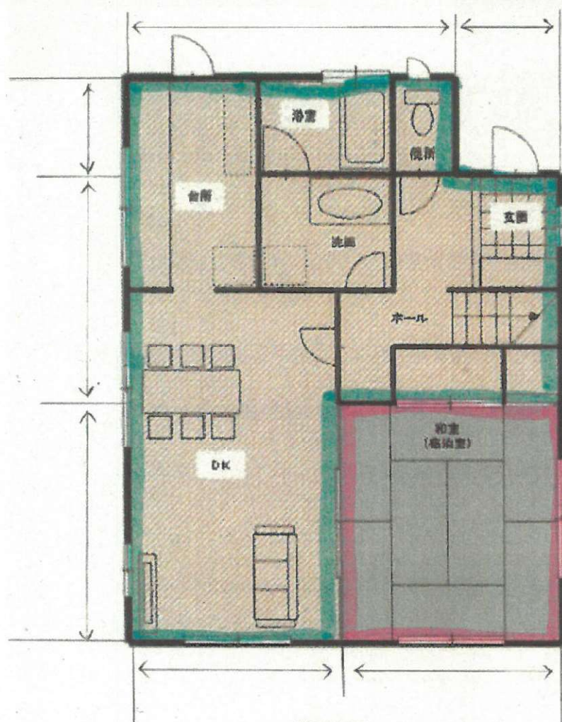
1階平面図
