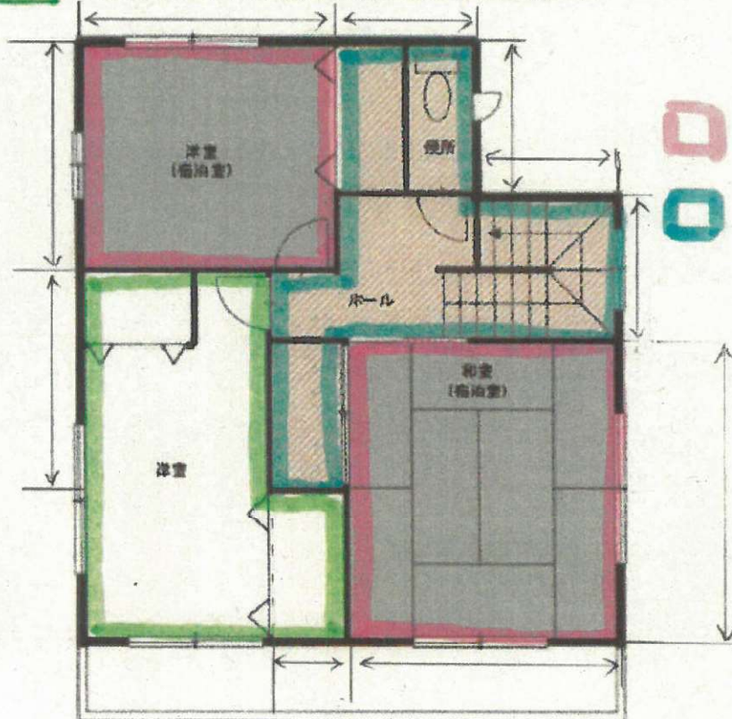
2階平面図
