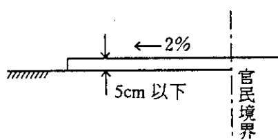
a—a' 断面図
