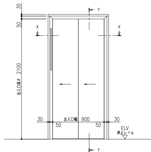
正面図（１：２０）
