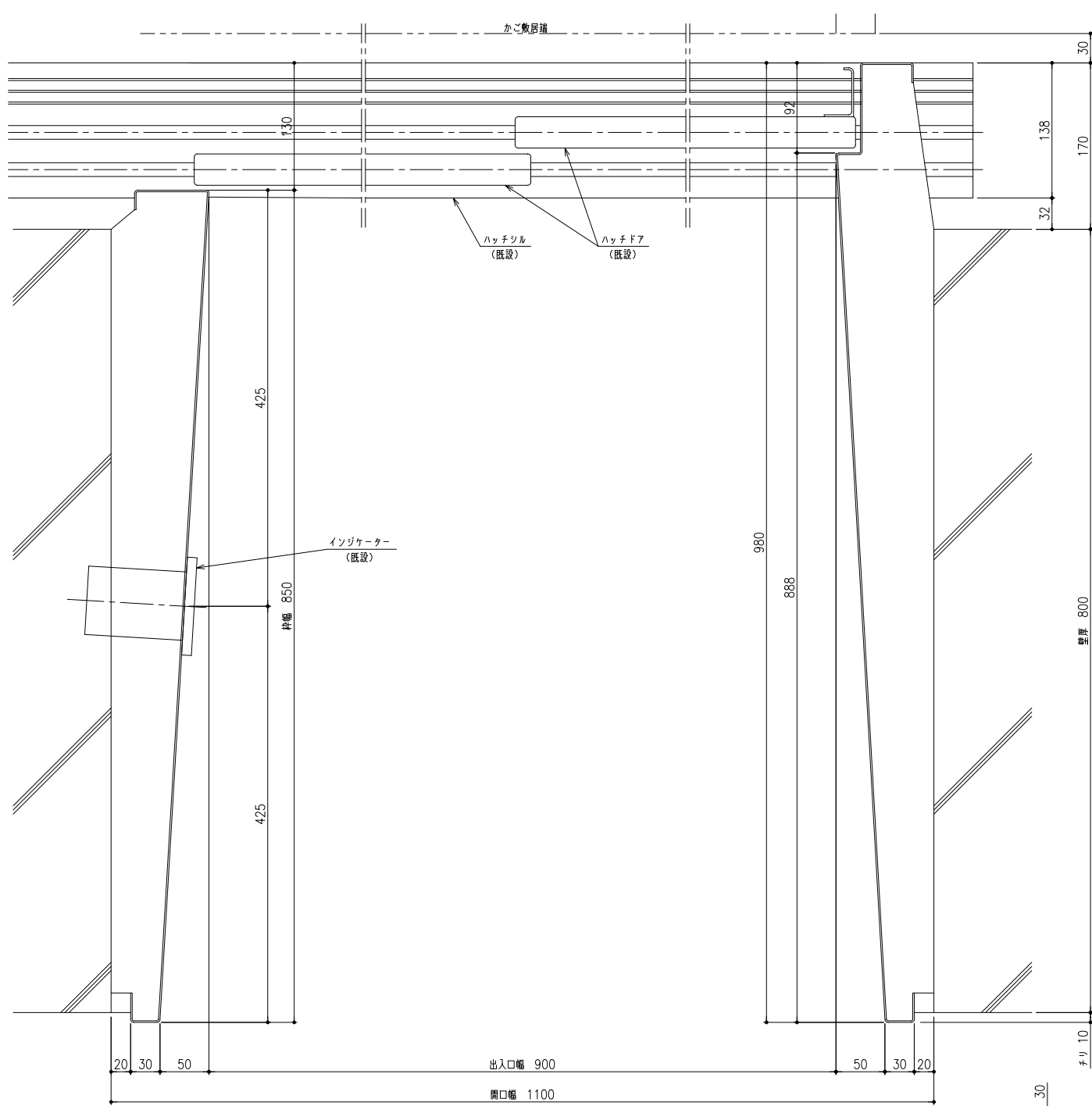
平面図〔断面XX〕（１：３）
