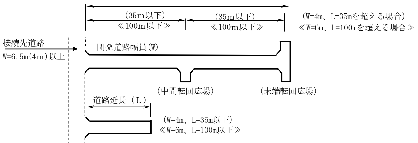
図 3 - 4 袋路状道路
