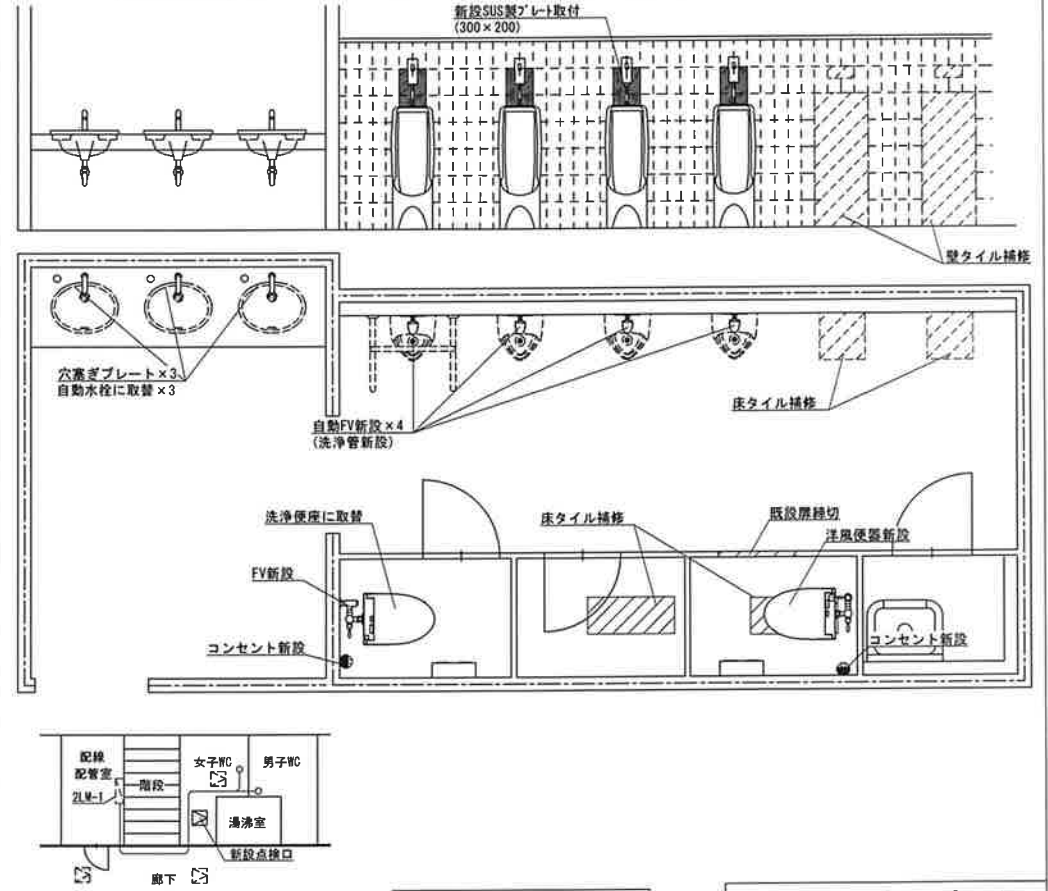
改修後 詳細図 1/40
