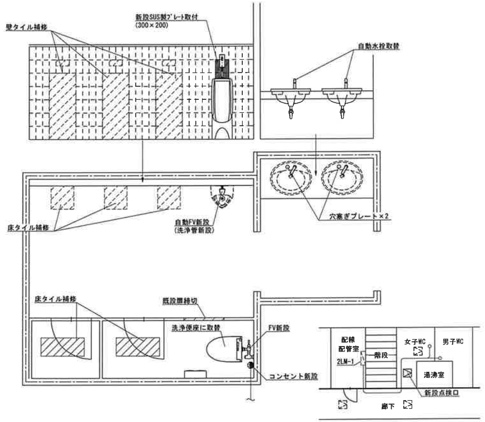
改修後 詳細図 1/40
