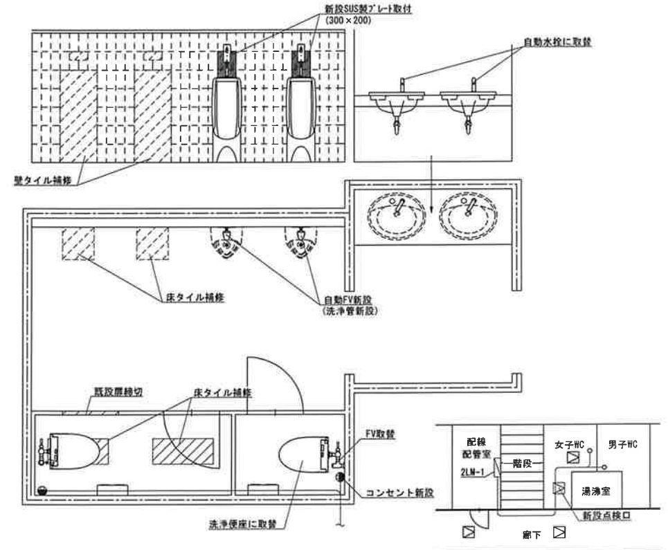
改修後 詳細図 1/40
