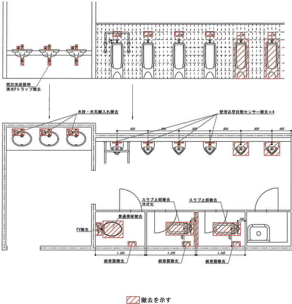
改修前 詳細図 1/40
