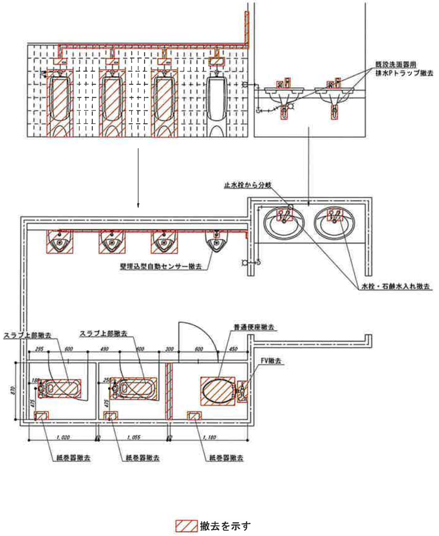
改修前 詳細図 1/40
