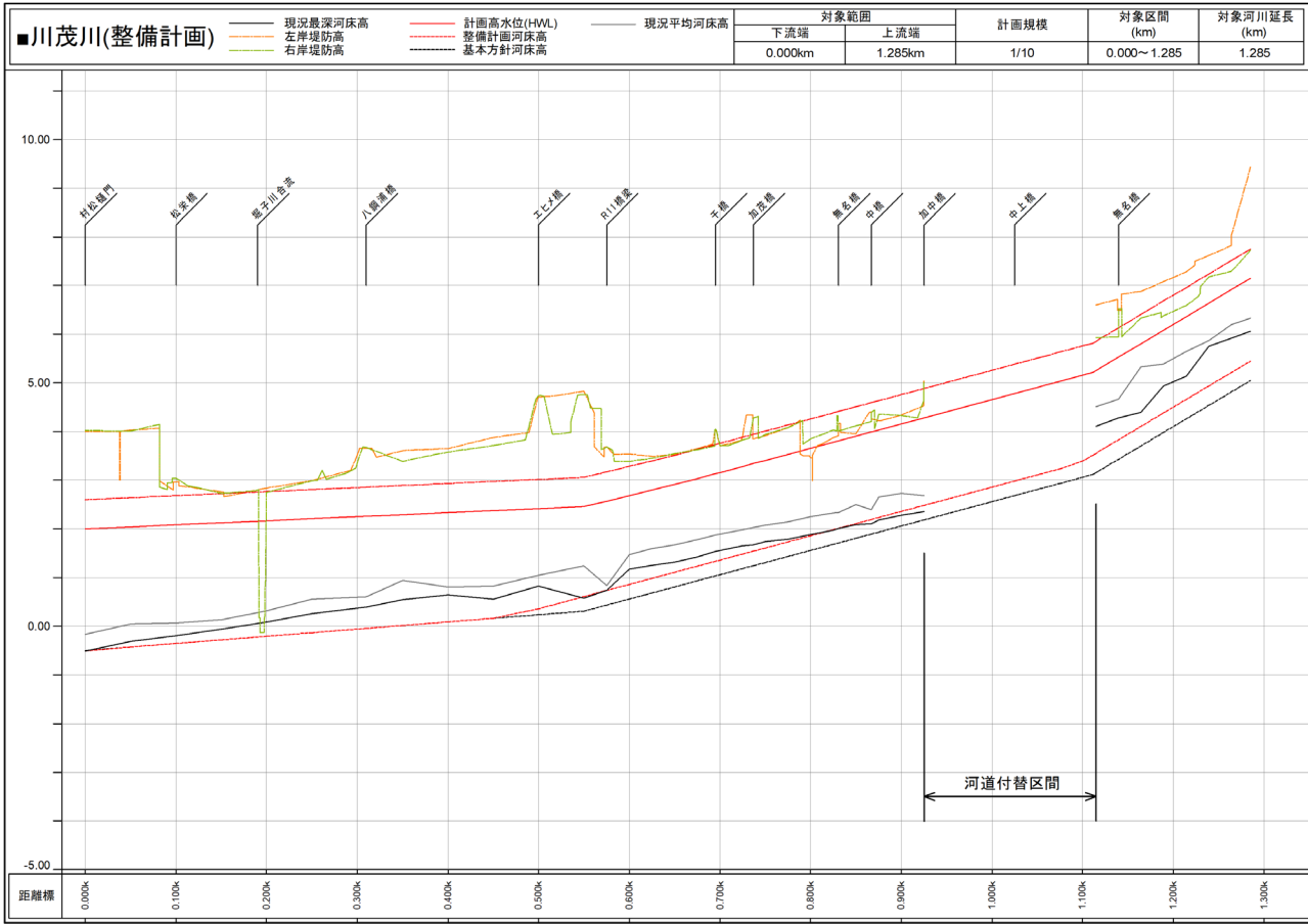
図 8 川茂川縦断面
