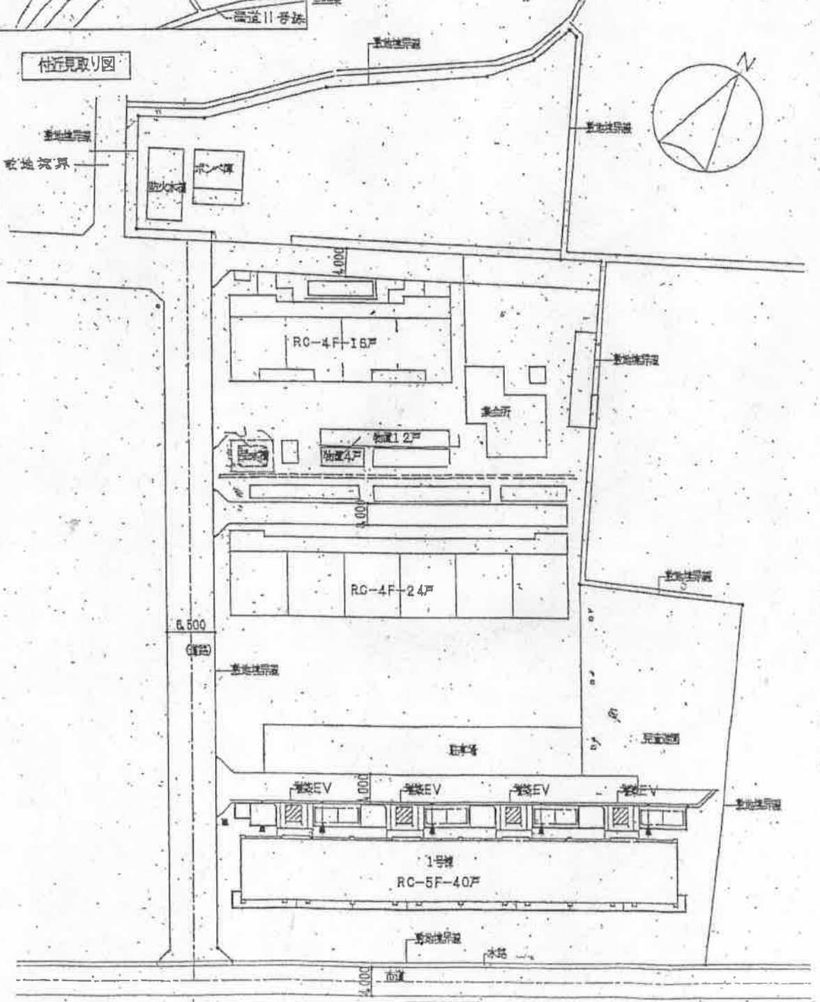
配置図
