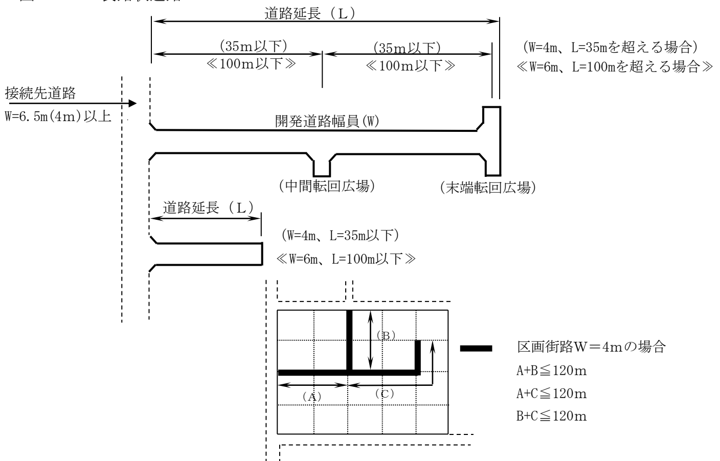
図 3 - 4 袋路状道路
