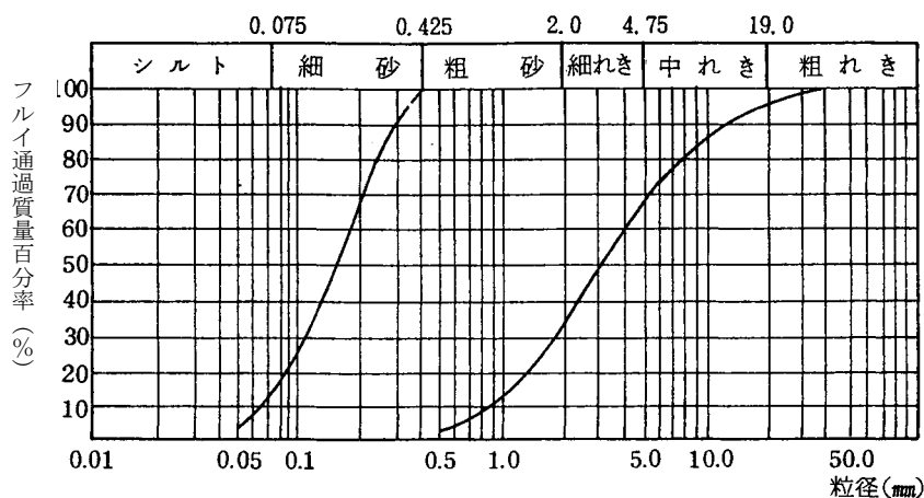
図8-2-1 使用砂の粒径加積曲線
