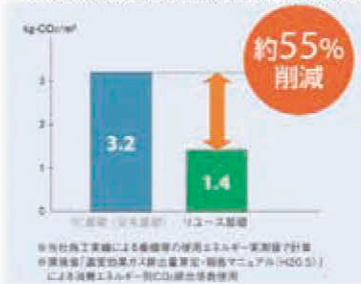
建設時の基礎工事におけるCO 2 排出量の比較
