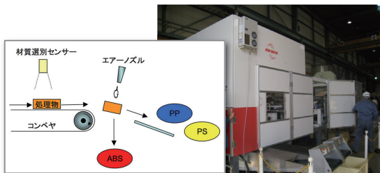
エアロソータⅢ(硬質ミックスプラスチック選別装置)
