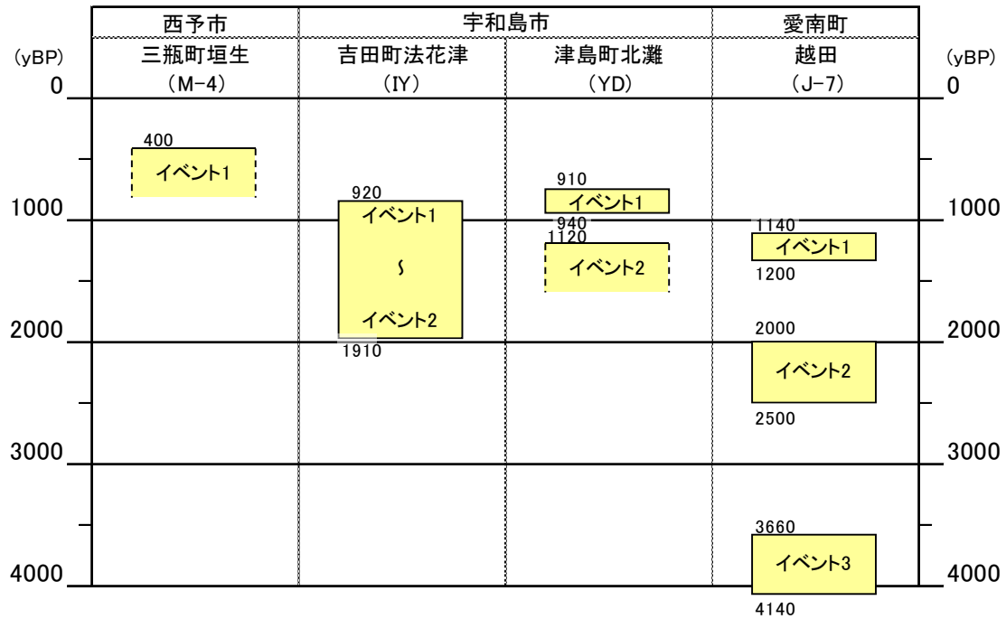
図-4.2.7 宇和海沿岸で推定される過去の津波イベント(1~3)
