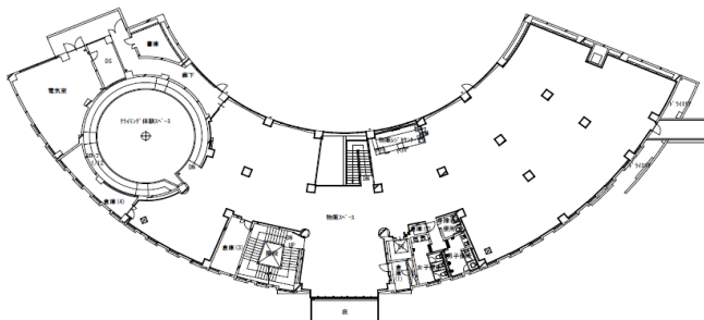
2階平面図
