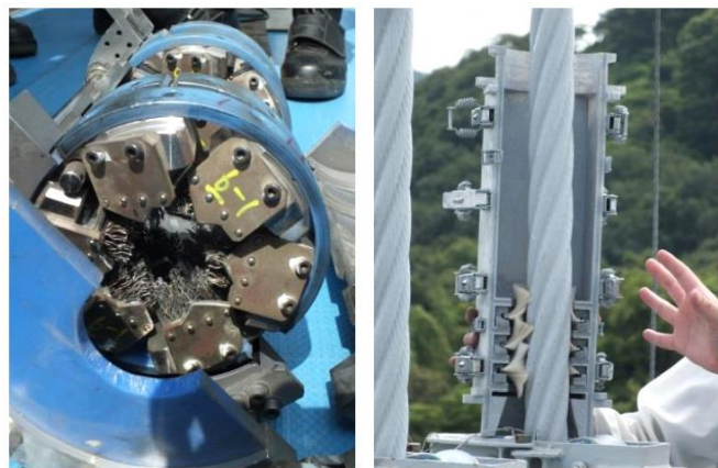
現場研修会：ハンガーロープ塗替塗装装置(因島大橋)
