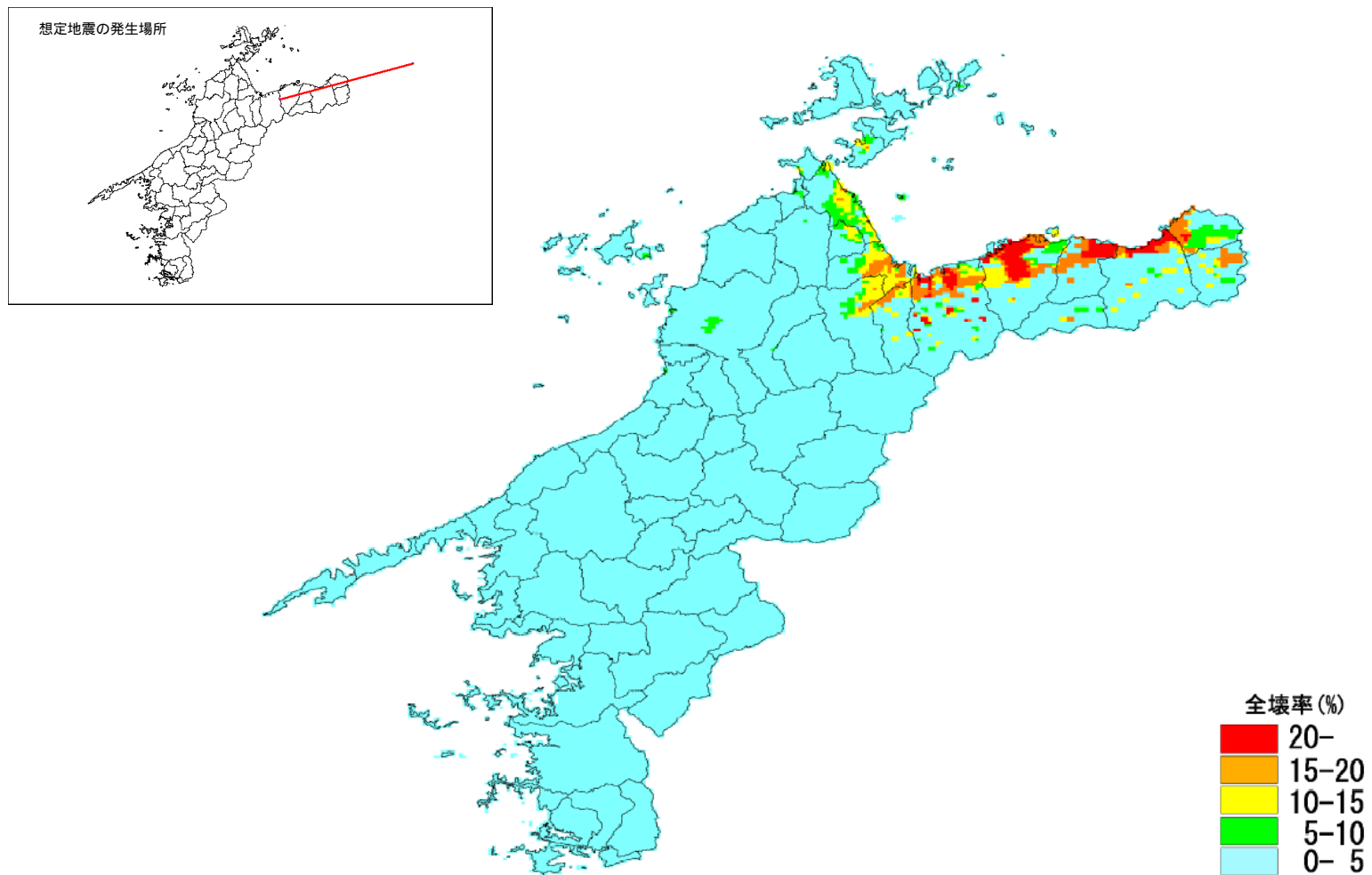
図2-3 揺れ・液状化による全建物の全壊率分布図（想定地震2）
