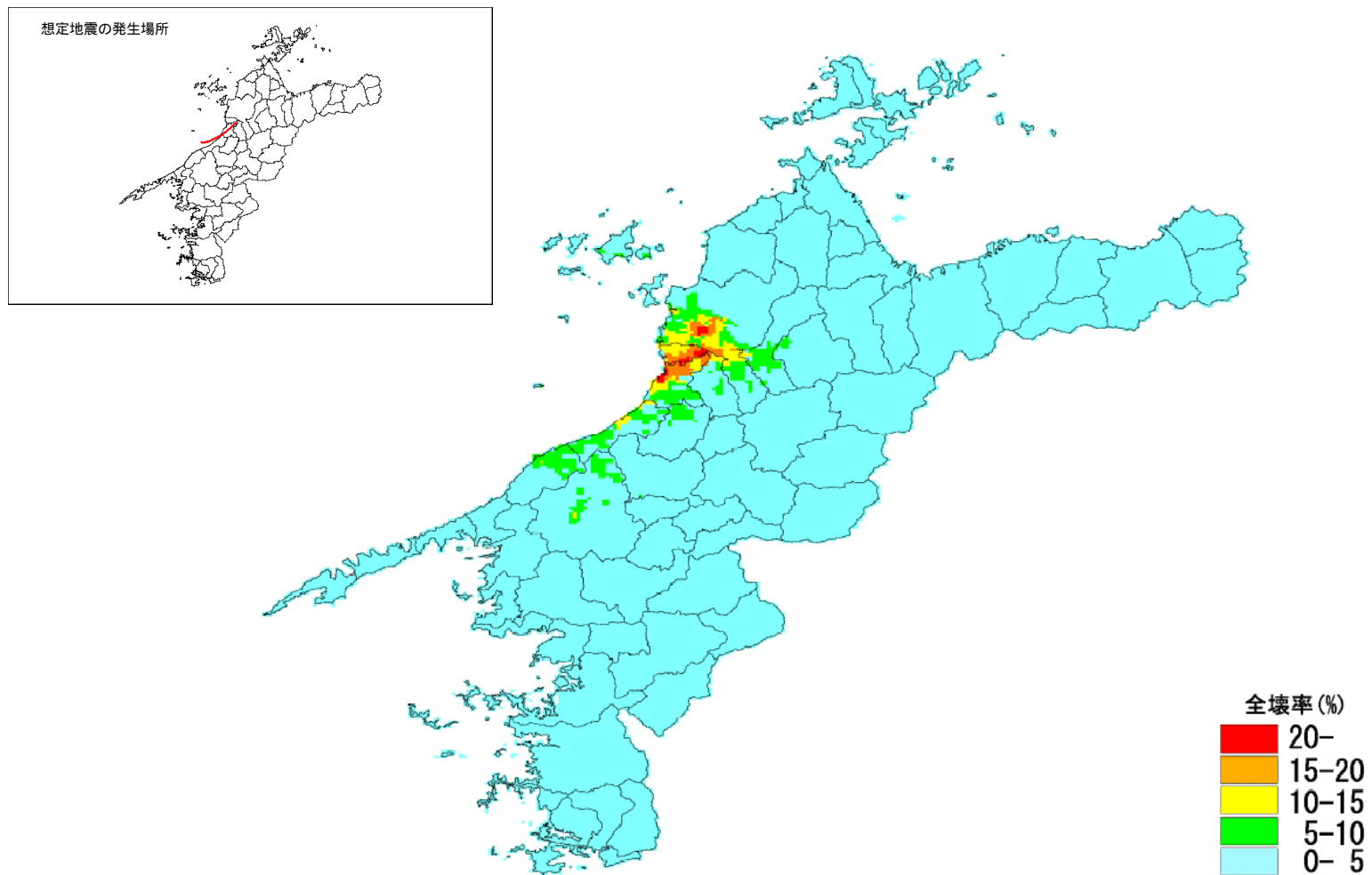
図2-4 揺れ・液状化による全建物の全壊率分布図 (想定地震3)
