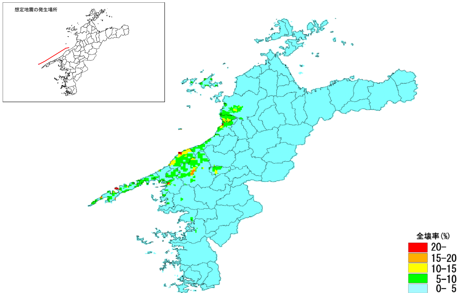
図2-5 揺れ・液状化による全建物の全壊率分布図（想定地震4）
