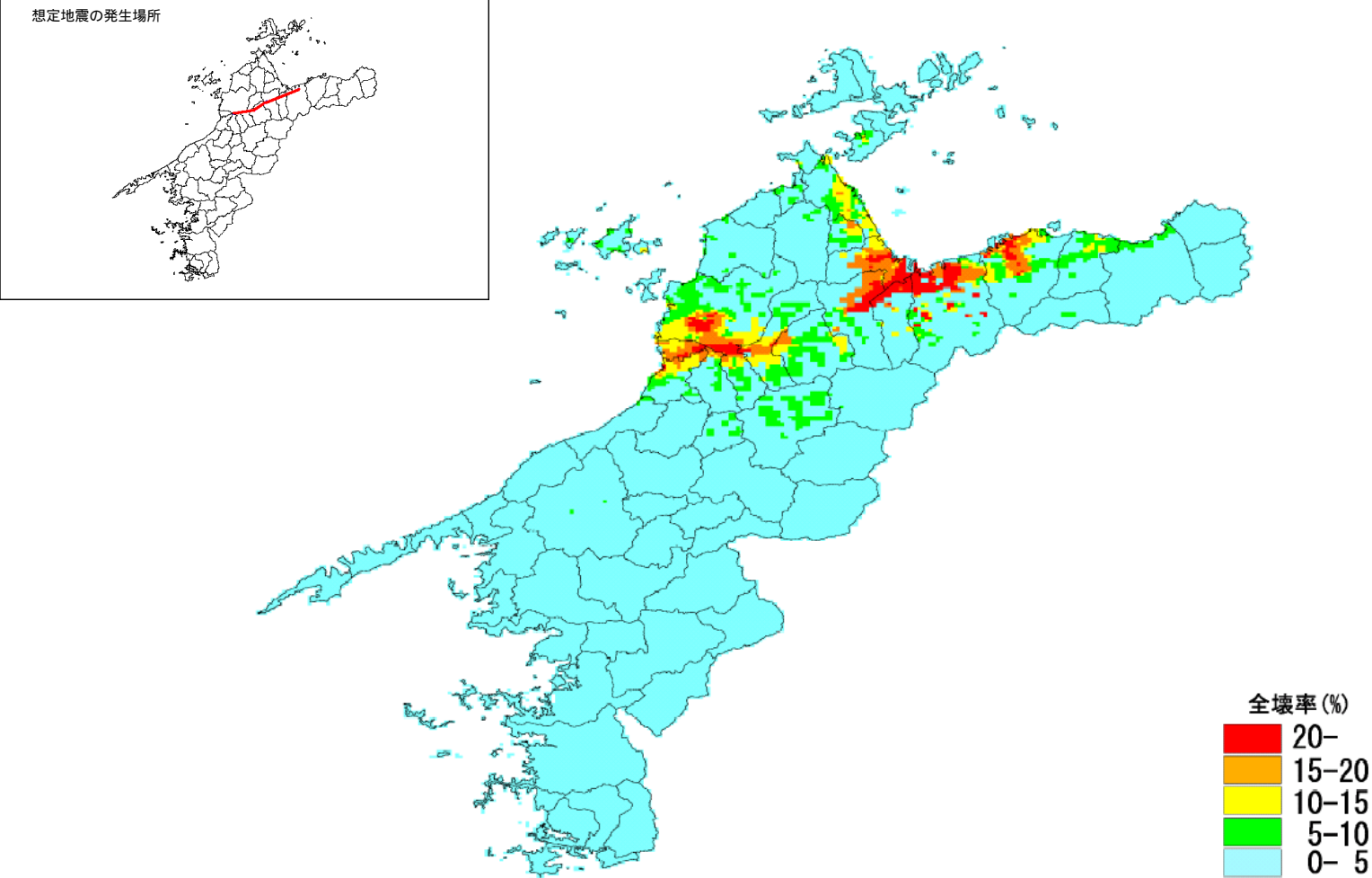
図2-2 揺れ・液状化による全建物の全壊率分布図 (想定地震1)
