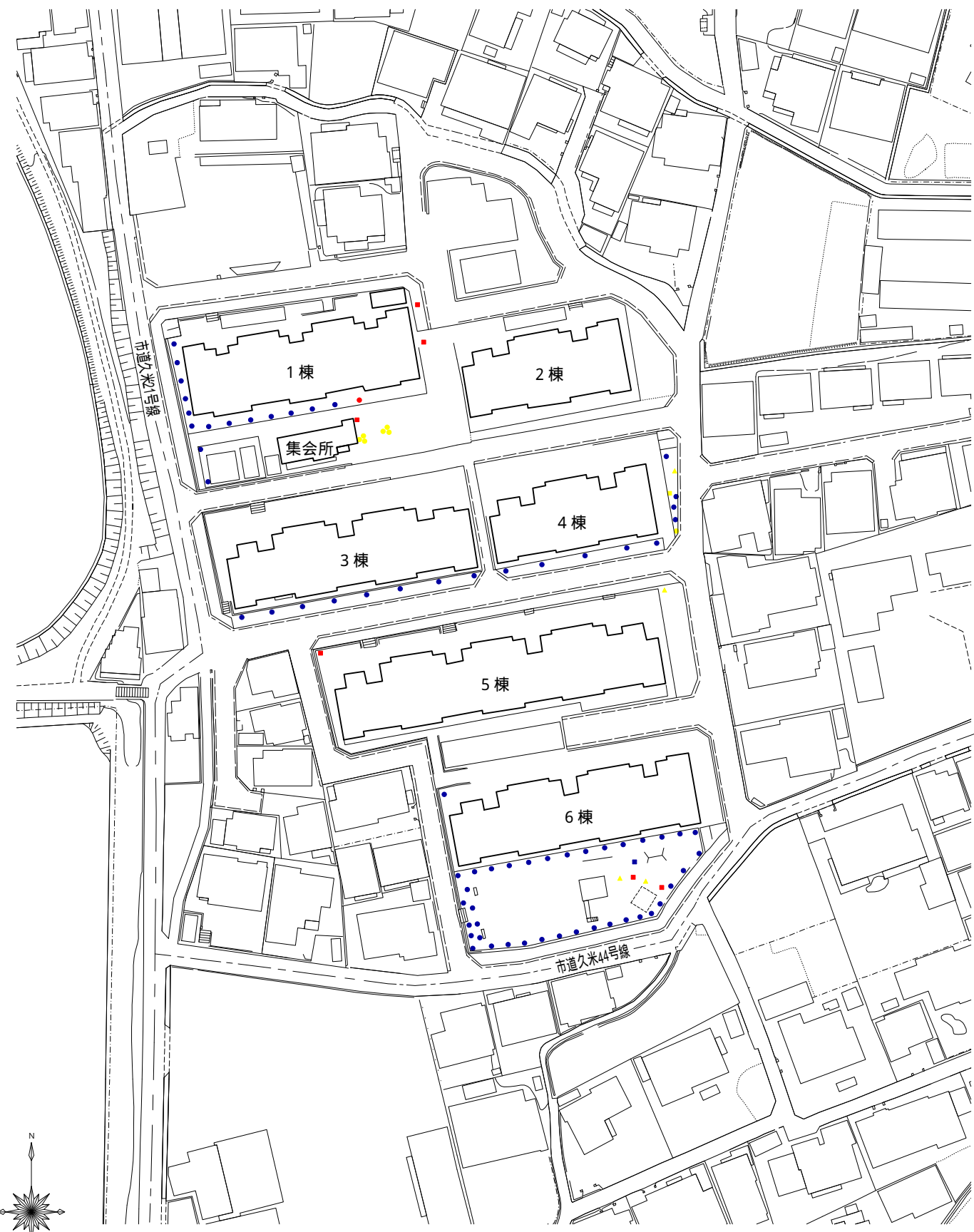
久米団地 配置図 NonScale
