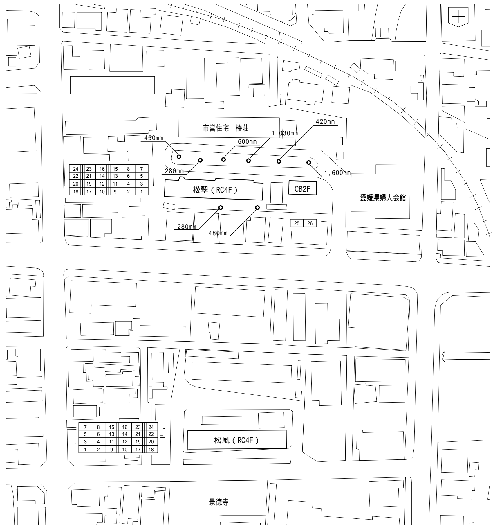
松風・松翠団地 配置図 NonScale
