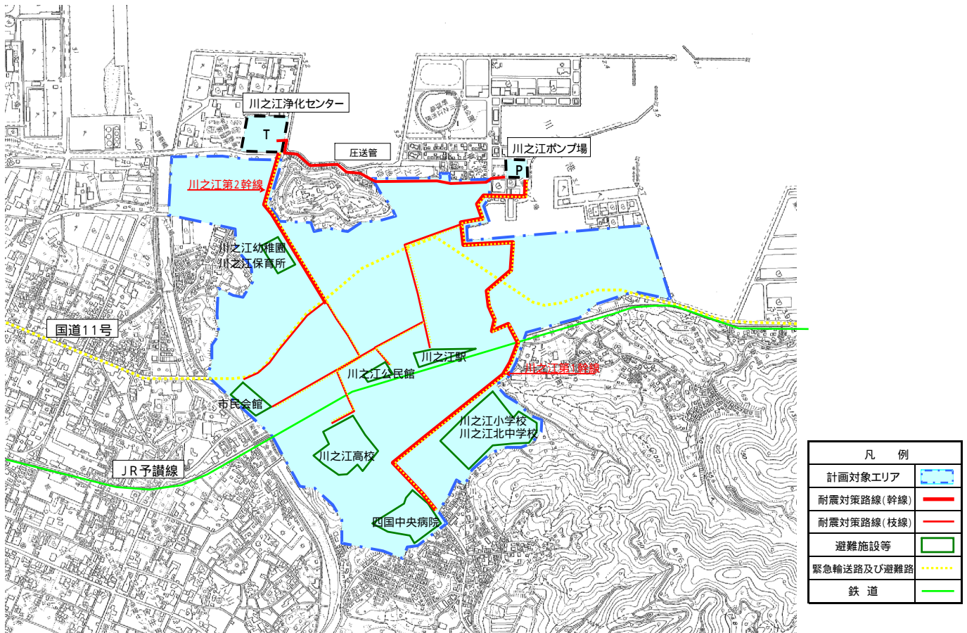
四国中央市下水道地震対策緊急整備計画図
